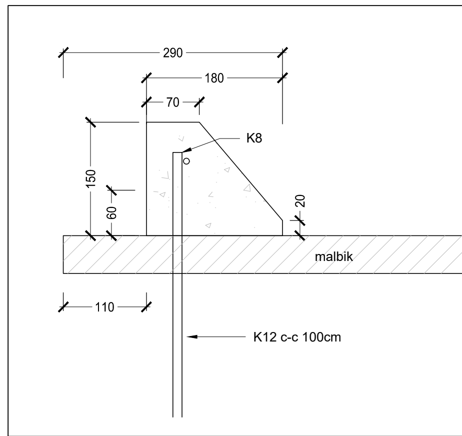
3.02 08 Kantsteinn 15cm, staðsteyptur Mkv. 1:5
