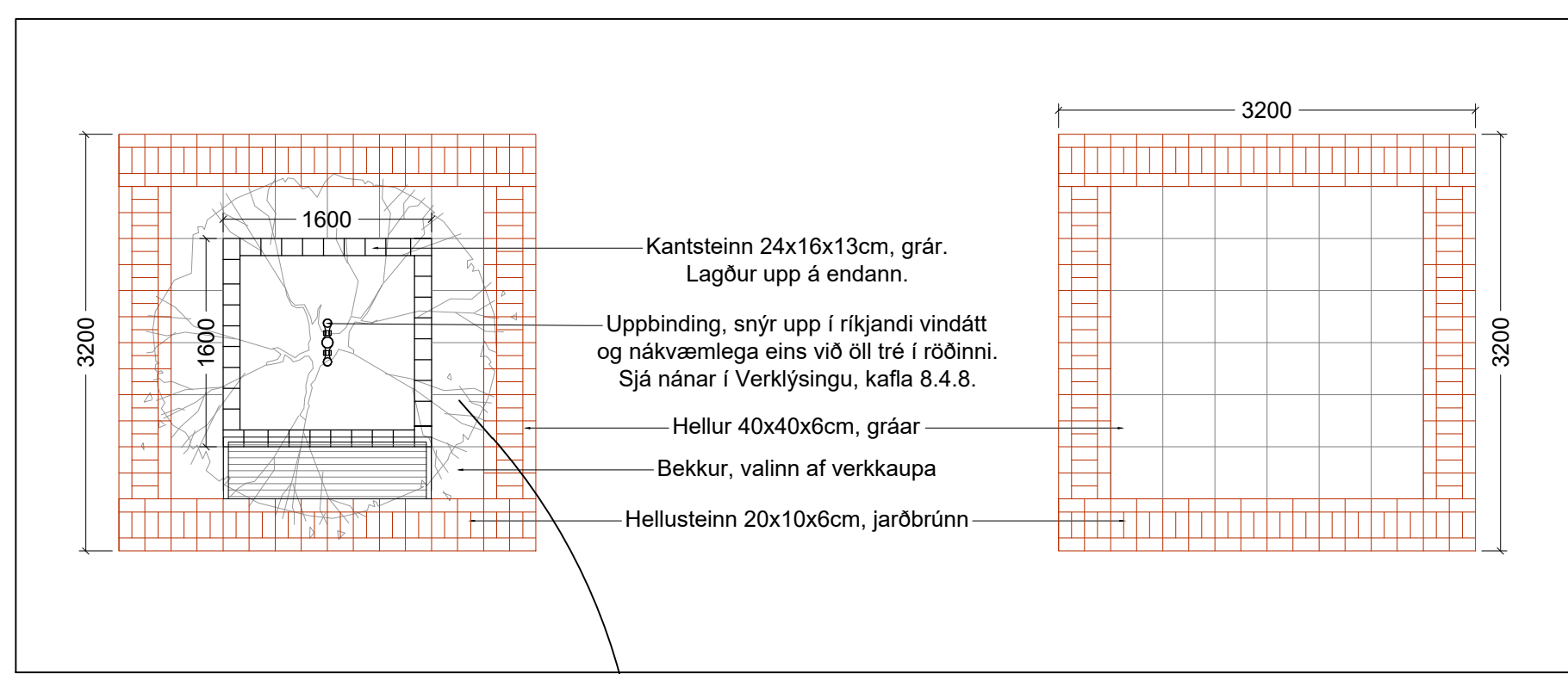
3.02 03 Hellumynstur á torgi Mkv. 1:50
