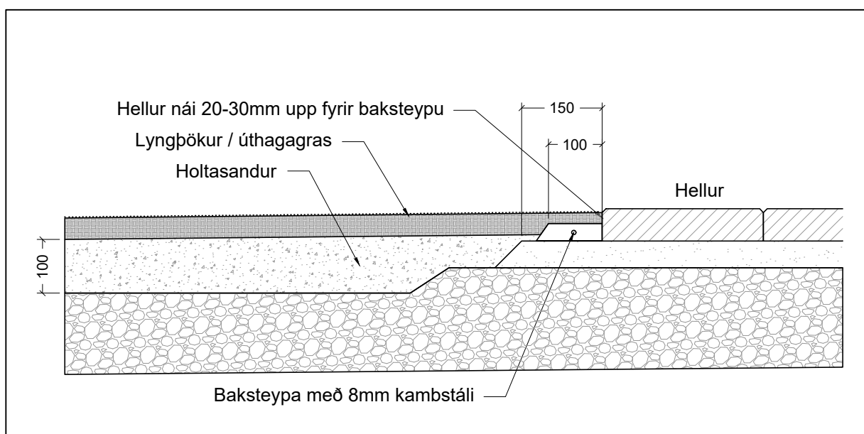
3.02 07 Almennur frágangur þar sem hellulögn liggur að grasi eða gróðursvæðum Mkv. 1:10
