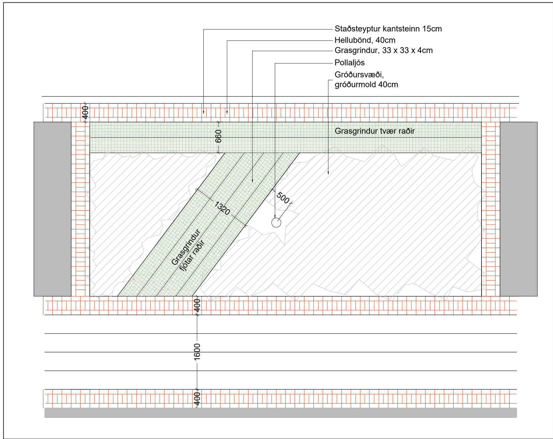
3.02 01 Grunnmynd, aðstæður á milli burðarbita meðfram vestur hlið húss Mkv. 1:50
