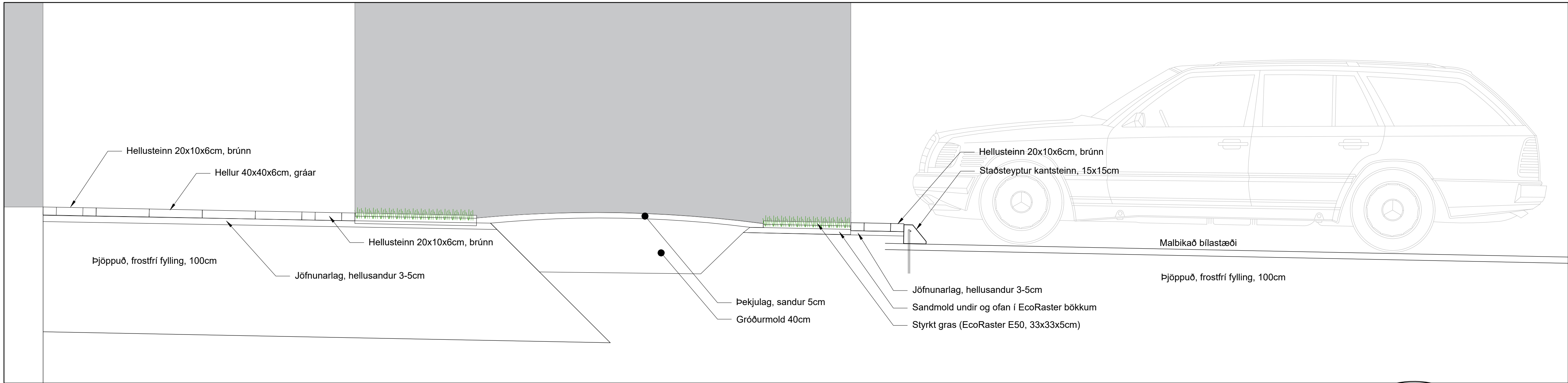
3.01 01 Snið - frágangur meðfram norðvesturhlöð Mkv. 1:20
