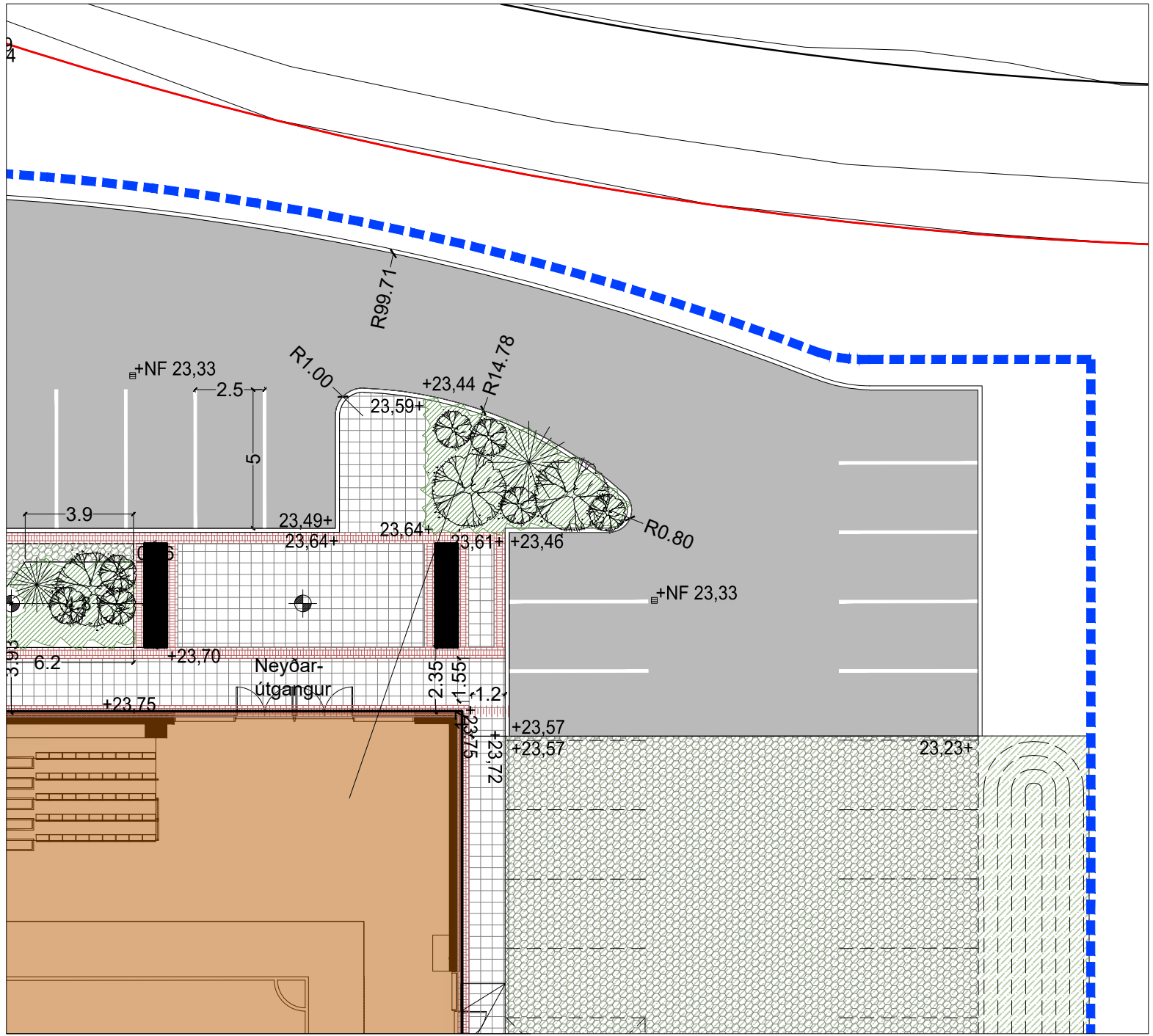
1.02 Málsetningar - norðurendi bílastæðis 02 Mkv. 1:200
