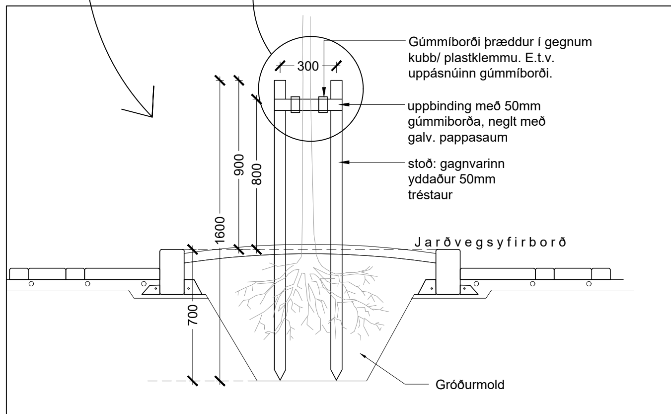
3.02 04 Trjáuppbindingar, grunnmynd og snið, sýnt í dæmigerðu beði á torgi Mkv. 1:20
