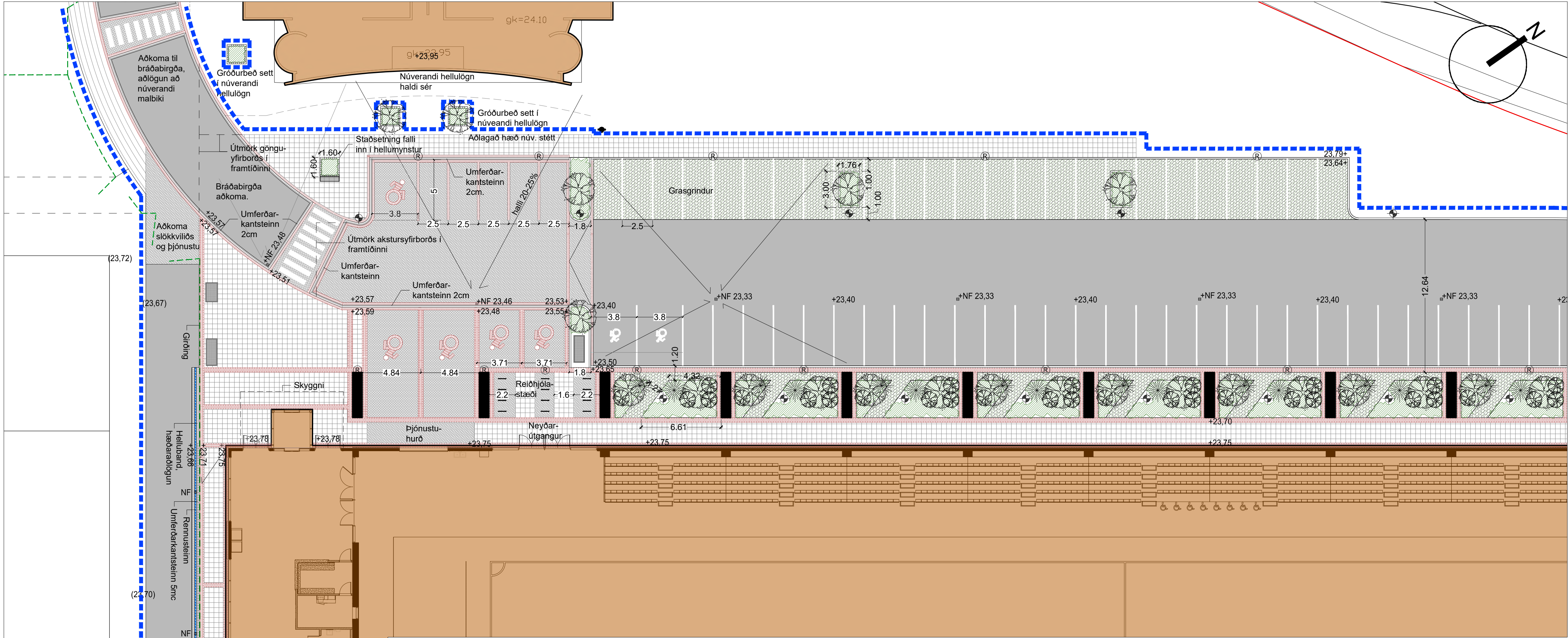
1.02 Málsetningar - Aðkoma og bílastæði 01 Mkv. 1:200
