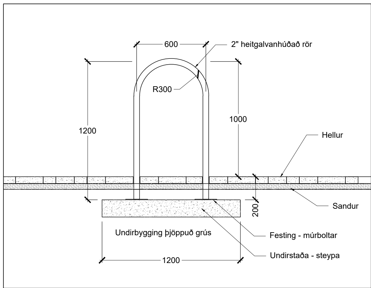
3.02 05 Hjólabogar, grunnmynd og snið Mkv. 1:20
