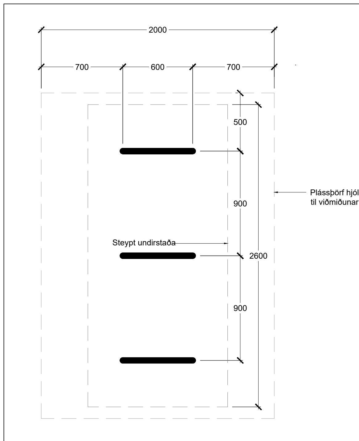
3.02 05 Hjólabogar, grunnmynd og snið Mkv. 1:20
