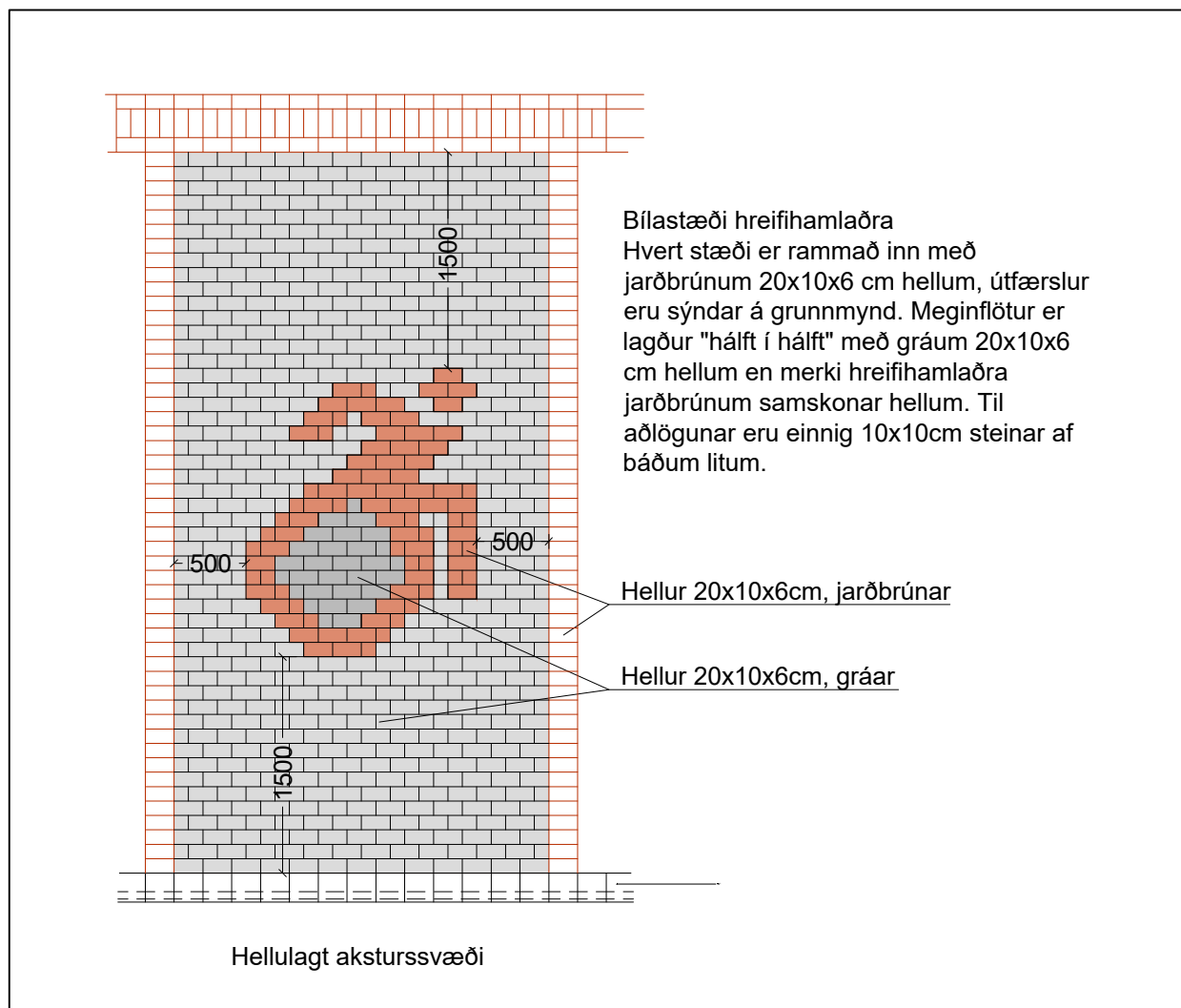
3.02 02 Frágangur á bilastæðum fyrir hreifhamlaða Mkv. 1:50
