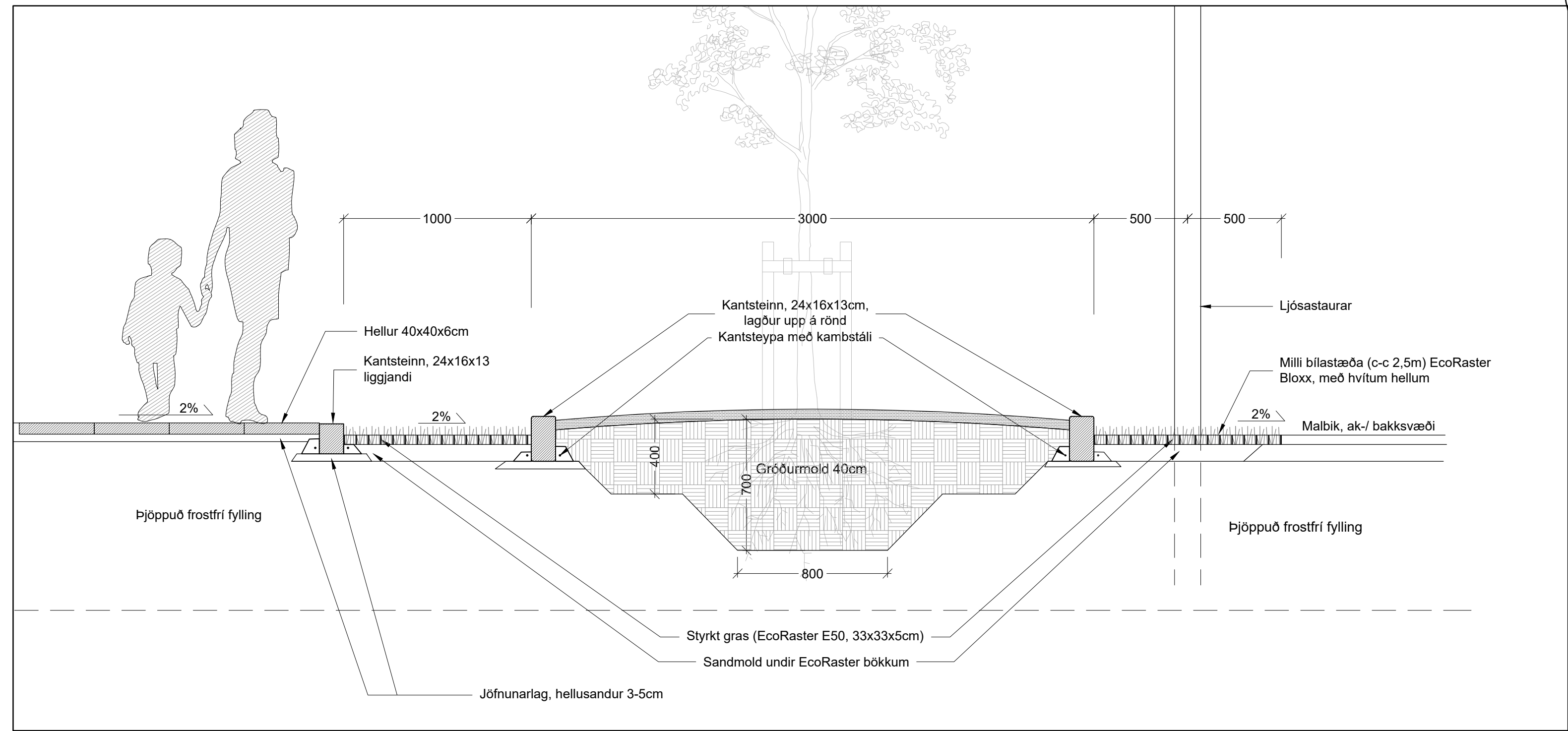
3.01 03 Uppbygging grænna bílastæða, gróðurbeða og aðliggjandi stéttar Mkv. 1:20
