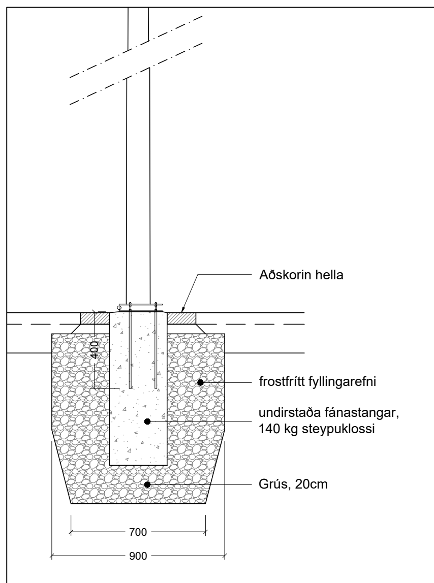
3.02 06 Fánastöng, undirstaða, almennur frágangur Mkv. 1:20
